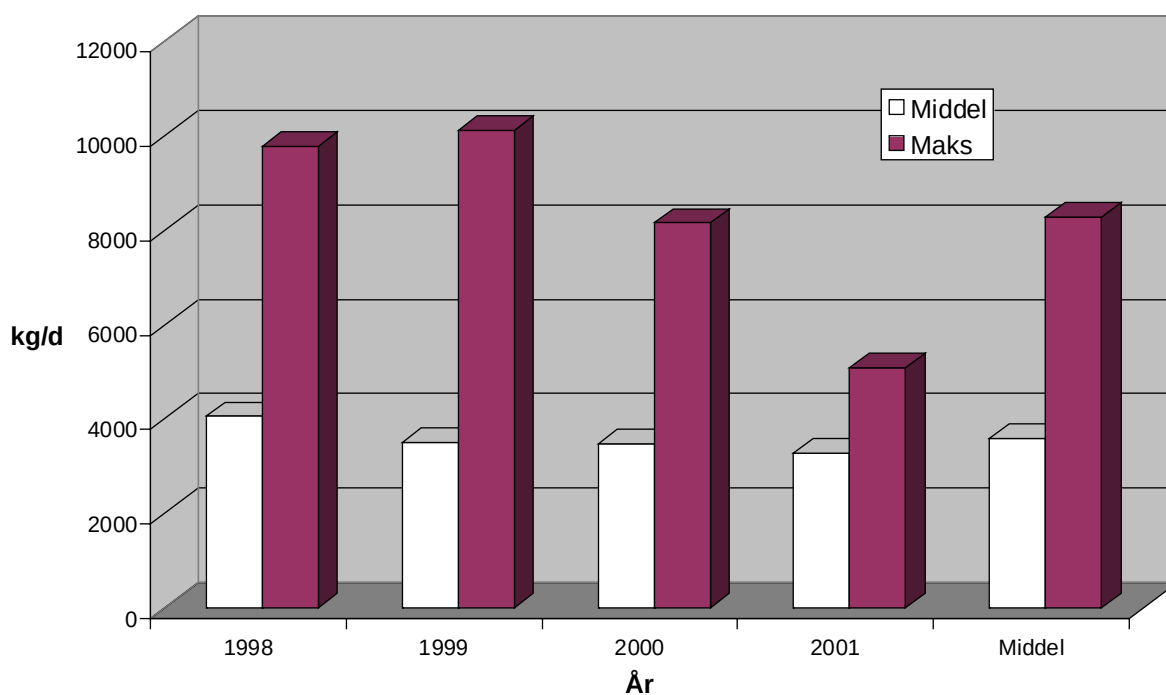
Figur 5. Tilførsel av \text{BOF}_7 på Øra renseanlegg 1998-2001.
