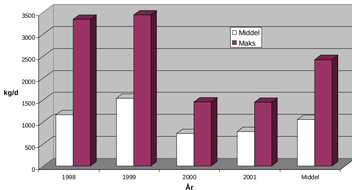
Figur 4. Tilførsler av \text{BOF}_7 til Nordre Follo renseanlegg i 1998-2001.
