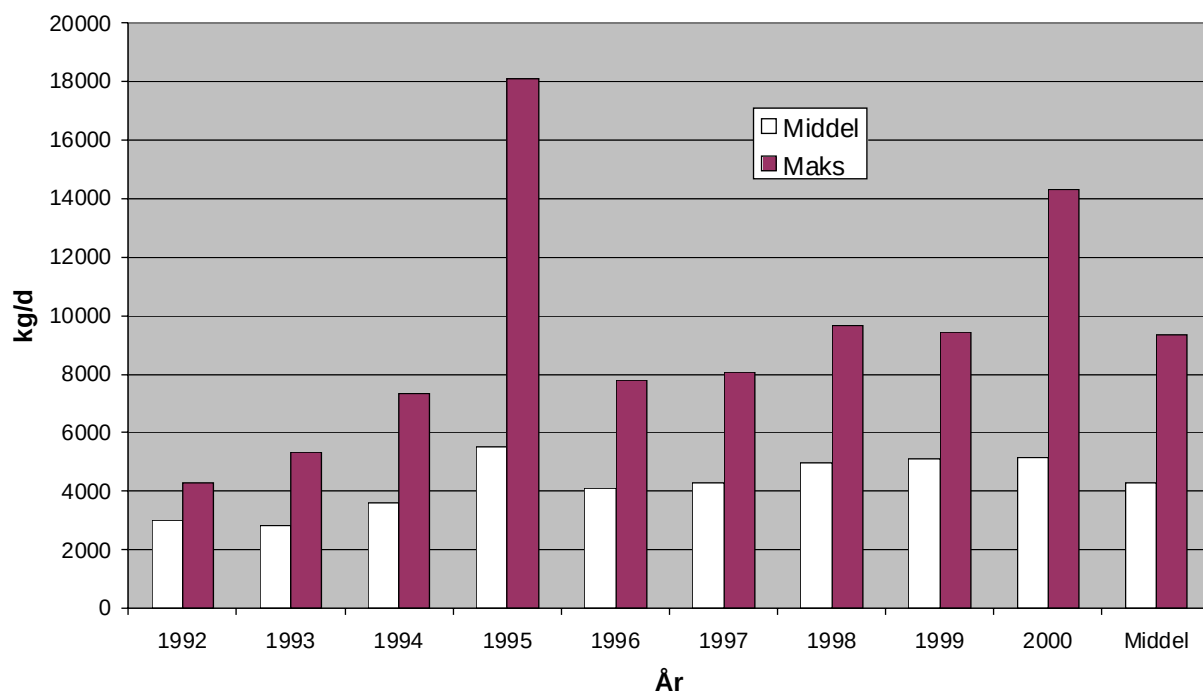
Figur 8. Tilførsel av KOF på Solumstrand renseanlegg 1992-2000.
