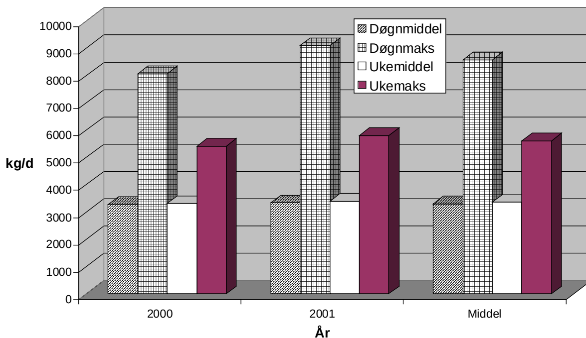
Figur 7. Tilførsel av KOF til Gardermoen renseanlegg i 2000 og 2001.
