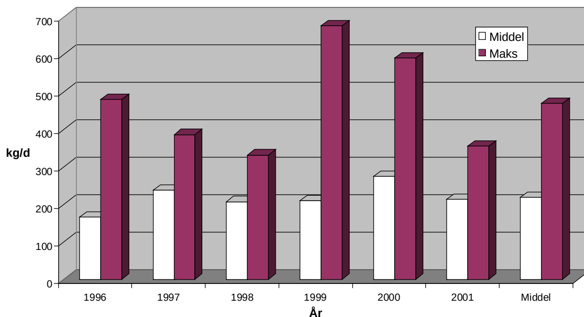
Figur 6. Tilførsel av \text{BOF}_7 til Oppdal renseanlegg i 1997-2001.
