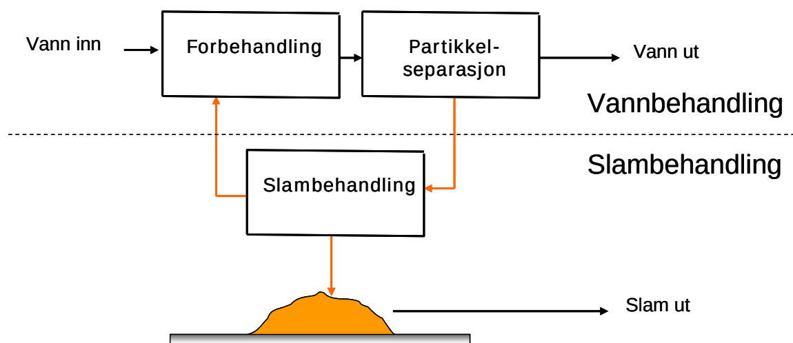
Figur 3.1 Oppbygging av primærrenseanlegg
