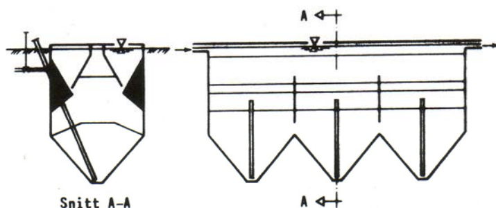
Figur 5.5 Sedimenteringsanlegg med integrert slamlager (Imhoff-tank)
