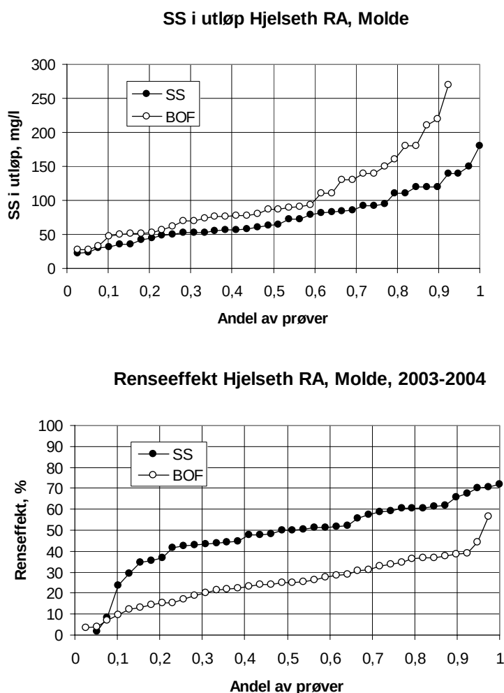
Figur 4.8 Renseresultater Hjelseth RA, Molde, 2003-2004. Finsilanlegg med 0,35 mm sil Dataene fra Hjelseth RA stammer fra blandprøver av 3-5 stikkprøver som er tatt over 1,5 – 5 timer på dagtid mens resultatene fra Elnesvågen er basert på døgnblandprøver.
