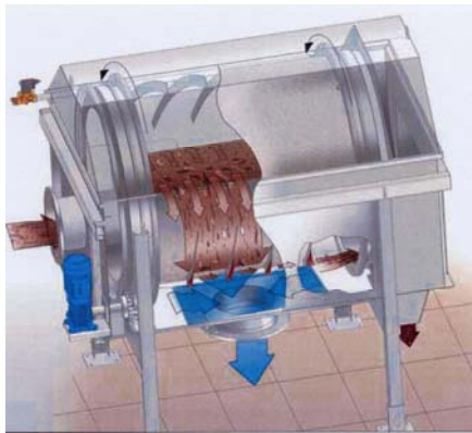
Figur 4.3 Eksempler på finsil av typen roterende trommelsil
