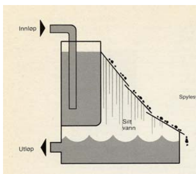
Figur 4.1 Stasjonære spaltesiler
