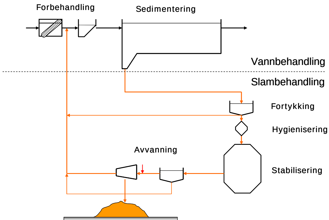
Figur 5.3 Oppbygging av tradisjonelt primærrenseanlegg basert på sedimentering og håndterings av slam i henhold til gjødselvareforskriften
