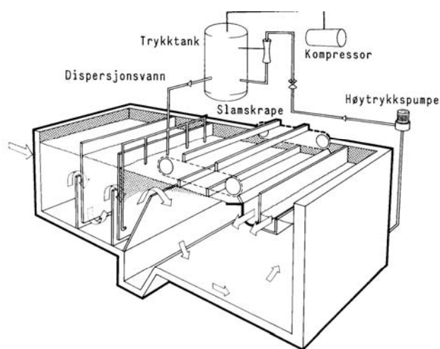
Figur 6.3 Flotasjonsanlegg.
