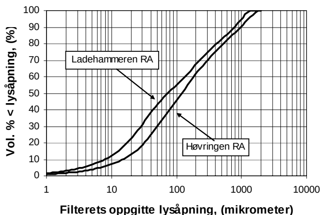
Figur 2.1 Partikkelstørrelsesfordelingen (vist som summasjonskurver) ved Høvringen og Ladehammeren renseanlegg i Trondheim i prøver tatt høsten 2004
