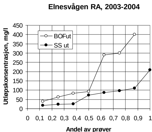
Figur 4.9 Renseresultater fra Elnesvågen RA i 2003-2004 (silåpning 0,35 mm)
