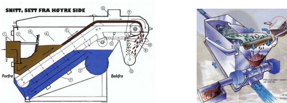
Figur 4.5 Eksempler på finsiler av typen roterende duksiler
