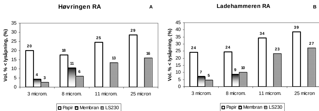
Figur 3. Sammenligning av resultatene fra membranfilter og papirfilter med partikkelstørrelsestetter (LS230) som gir volum % mindre enn lysåpningen. Figur 3A og B viser resultater fra henholdsvis Høvringen og Ladehammeren RA.
