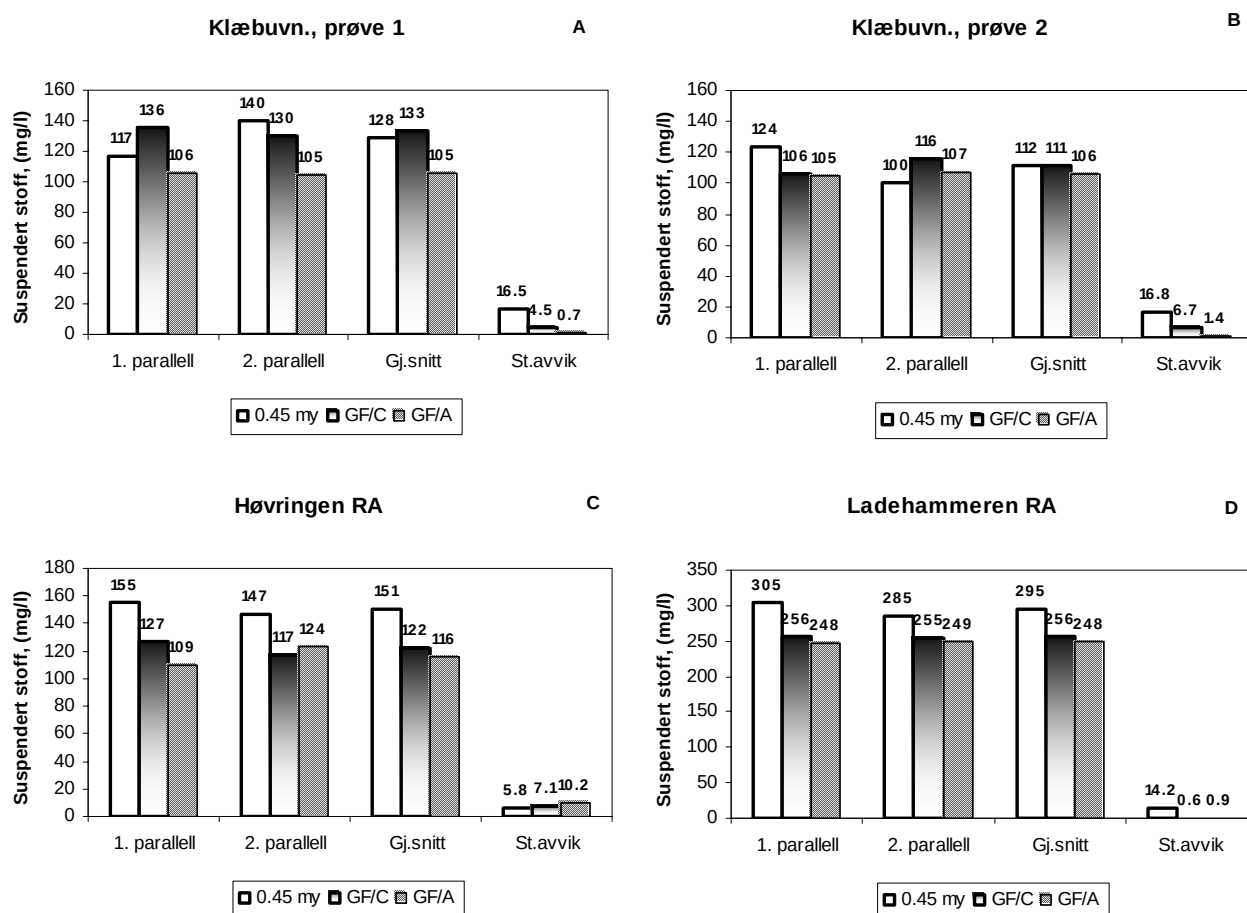
Figur 2. Sammenligning av 0.45 µm membran-, GF/C- og GF/A-filter. Figur 2A og B er med avløpsvann fra vår forsøkshall i Klæbu, Trondheim og Figur 2C og D er med avløpsvann fra henholdsvis Høvringen og Ladehammeren renseanlegg i Trondheim. Figurene viser resultatene fra 2 paralleller, gjennomsnitt av disse og standardavviket. Tallverdiene er angitt over søylene i figurene.
