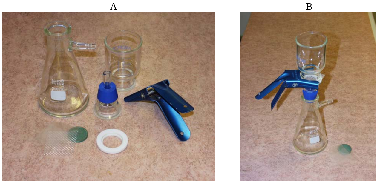
Figur 1. Filteroppsats benyttet under forsøkene. Figur 1A viser de enkelte delene og eksempler på nylonnett som ble benyttet. Figur 1B viser oppmontert filteroppsats med nylonnett. Merk at silen i filteroppsatsen (rund grønn sil) ikke ble benyttet sammen med nylonnett.
