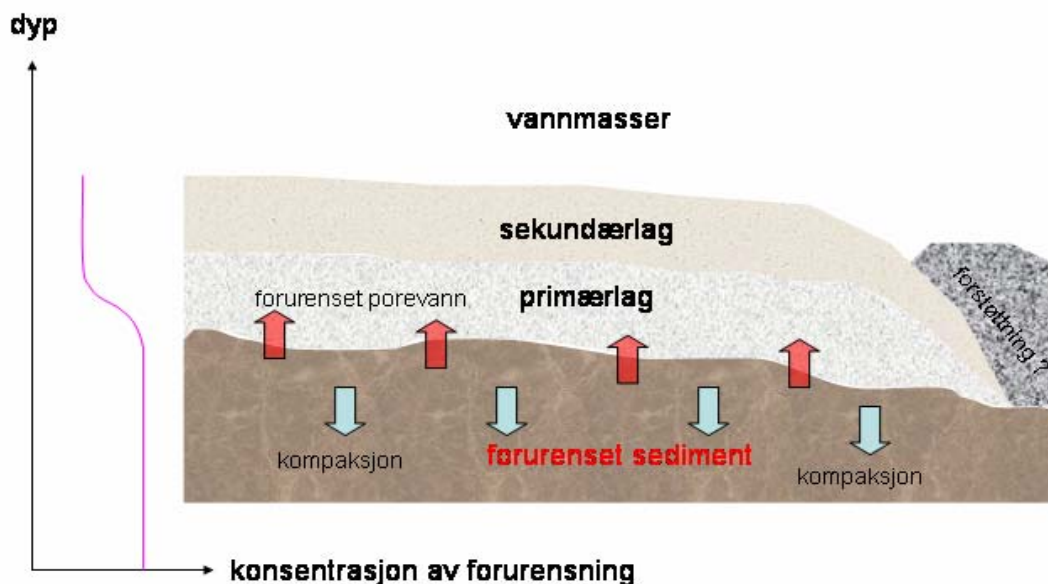
Figur 3. Overlagring av bløte sedimenter reduserer porevolumet. Denne prosessen – kompaksjon – fører enten til overtrykk eller porevannsutstrømning. Overtrykk er uønsket i denne sammenhengen. Forurensset porevann vil trenge opp i tildekkingsedimentene, men uten å komme i kontakt med vannmassene ovenfor. Konsentrasjon av forurensset stoff avtar med tykkelsen på tildekkingsmassene. I enkelte tilfeller kan det være aktuelt med to tildekkingslag, et primærlag og et sekundærlag, enten for å lage en barriere eller for å stabilisere primærlaget. Geomembraner og forstøttinger omhandles ikke i denne rapporten, men kan være viktig ved vurderingen av hvilke tildekkingsmasser som er optimale.
