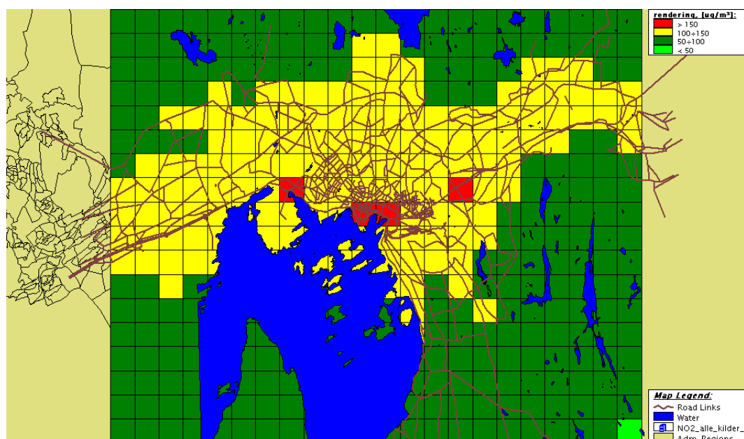
Figur A6: Niende høyeste timeverdi for \text{NO}_2 i perioden 01.01.01 – 30.04.01 og 01.10.01 – 31.12.01
