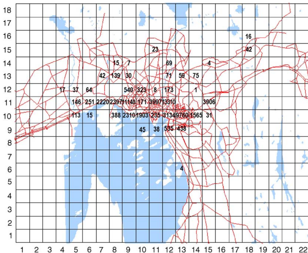
Figur 6: Antall personer utsatt for overskridelser av nasjonale mål i 1998 av \text{NO}_2 i felt og bygning konvertert til felt.
