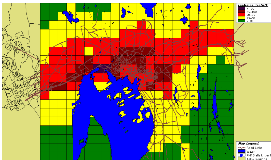
Figur A1: Åttende høyeste døgnverdi for PM 10 i perioden 01.10.95 – 31.03.96
