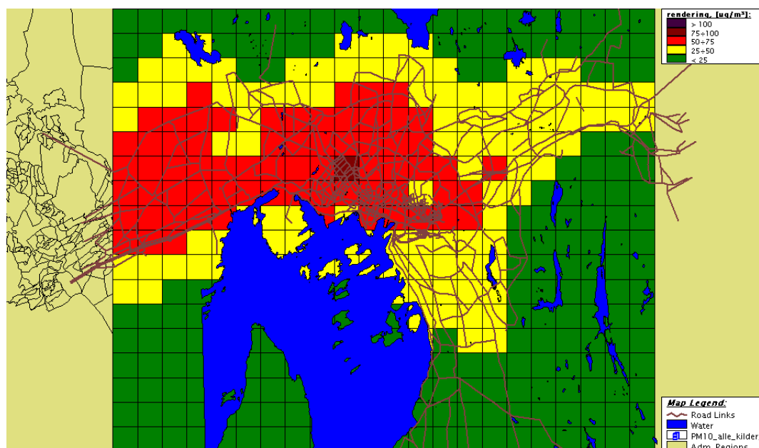
Figur A5: Åttende høyeste døgnverdi for \text{PM}_{10} i perioden 01.01.01 – 30.04.01 og 01.10.01 – 31.12.01
