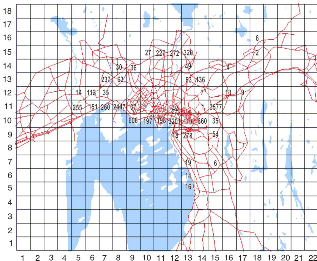
Figur 8: Antall personer utsatt for overskridelser av nasjonale mål i 2001 av \text{NO}_2 i felt og bygning konvertert til felt.
