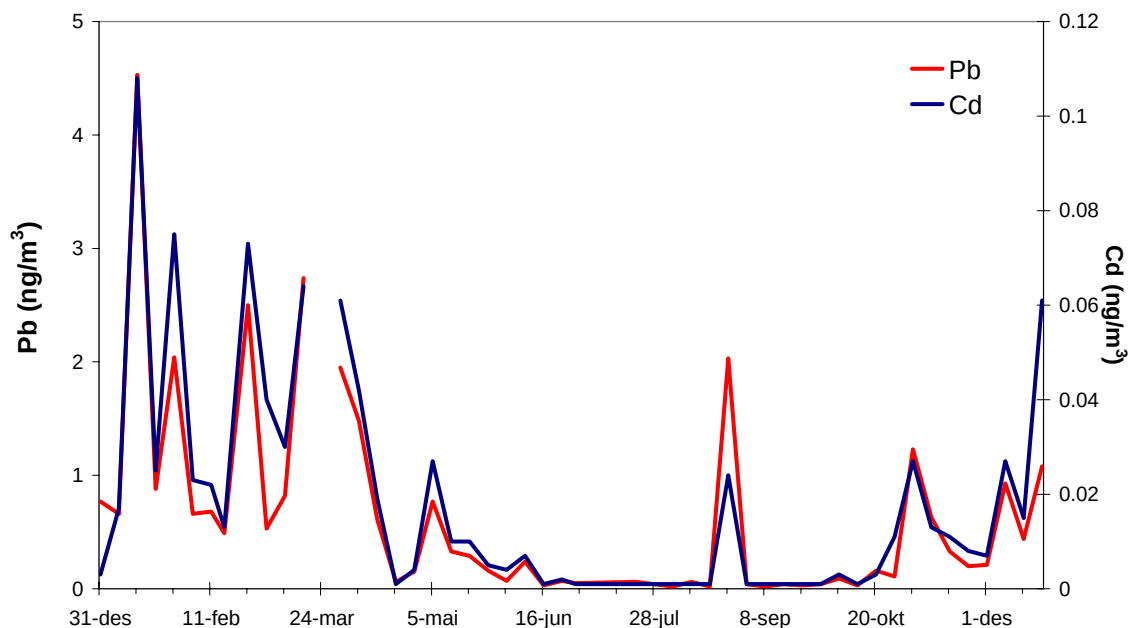
Figur 5.10: Ukentlige luftkonsentrasjoner av bly og kadmium på Zeppelinfjellet i 2004. Enhet: ng/m 3 .
