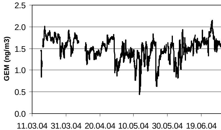
Figur 5.12: Tidsserier for elementært kvikksølv i gassfase (GEM) ved Zeppelin, våren 2004.
