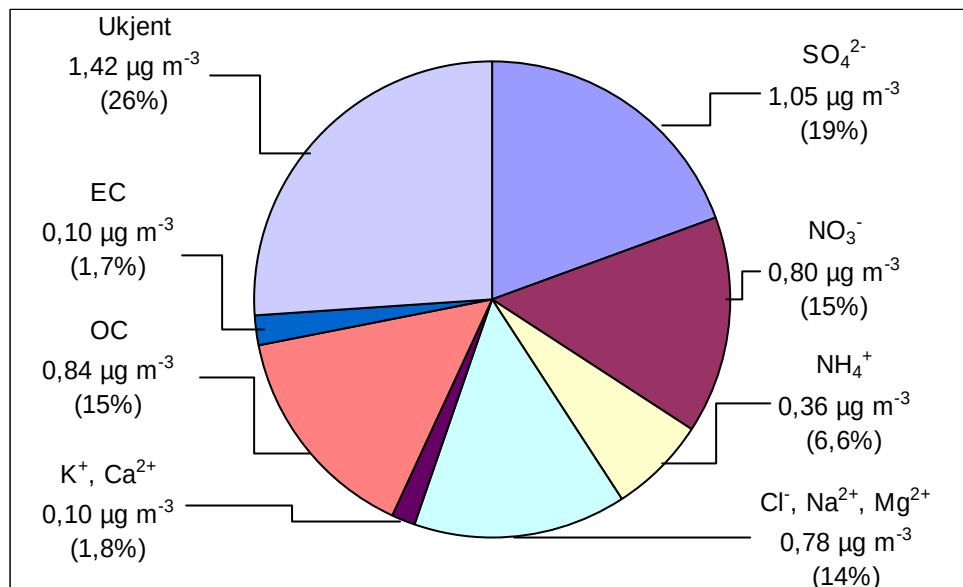
Figur 6.2: Gjennomsnittlig kjemisk sammensetning av partikler (massebalanse) i \text{PM}_{10} -fraksjonen på Birkenes i perioden 01.01.04-31.12.04. Gjennomsnittlig massekonsentrasjon av \text{PM}_{10} er 5,4 \mu\text{g m}^{-3} .
