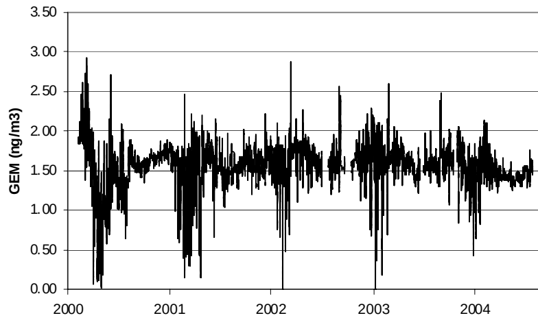
Figur 5.11: Tidsserier for elementært kvikksølv i gassfase (GEM) ved Zeppelin, 2000-2004.
