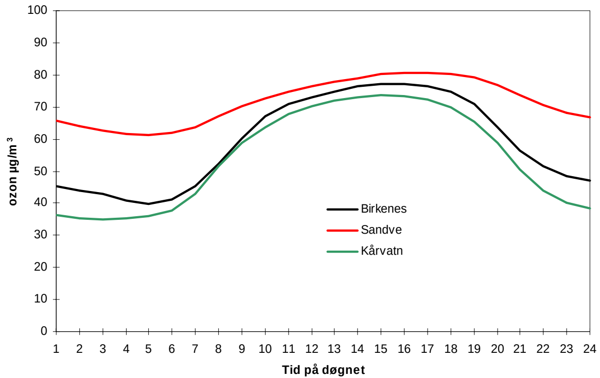
Figur 4.5: Midlere døgnvariasjon av ozon ( \mu\text{g}/\text{m}^3 ) for Birkenes, Sandve og Kårvatn, april-september 2004.
