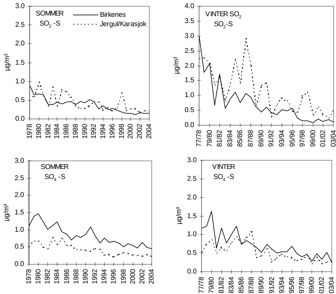
Figur 3.8: Middelkonsentrasjoner av partikulært sulfat og svoveldioksid i luft for vinterhalvårene 1977/1978 – 2003/2004 (oktober-mars) og sommerhalvårene 1978–2004 på Birkenes og Jergul/Karasjok.
