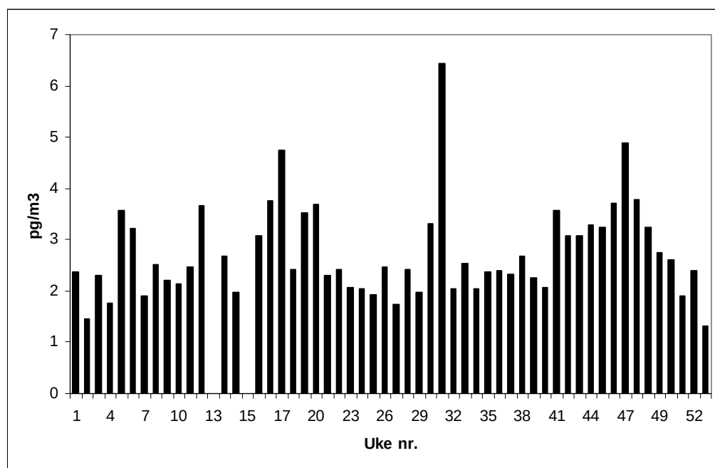
Figur 5.15: Ukentlig luftkonsentrasjon av \gamma -HCH på Zeppelinfjellet i 2004. I en del tilfeller ble flere målinger gjort i løpet av en uke. I slike tilfeller ble prøvene nummerert med ukenummer og en bokstav, f.eks. 14a og 14b.
