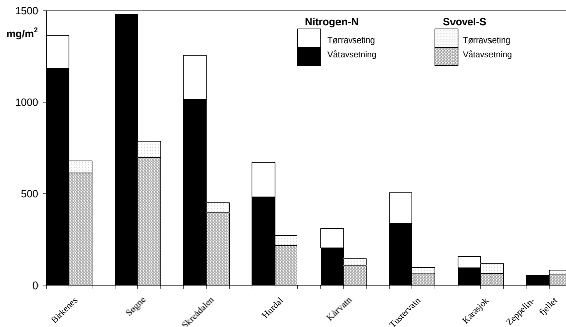
Figur 3.2: Total avsetning (våt- og tørravsetning) av svovel-S ( \text{SO}_2 , \text{SO}_4^{2-} ) og nitrogen-N ( \text{NO}_2 , \text{NH}_4^+ , \text{NH}_3 , \text{NO}_3^- , \text{HNO}_3 ) på norske bakgrunnsstasjoner, 2004.
