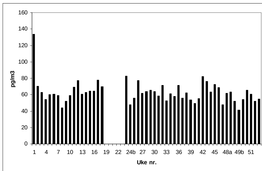
Figur 5.7: Ukentlig luftkonsentrasjon av HCB på Birkenes i år 2004.
