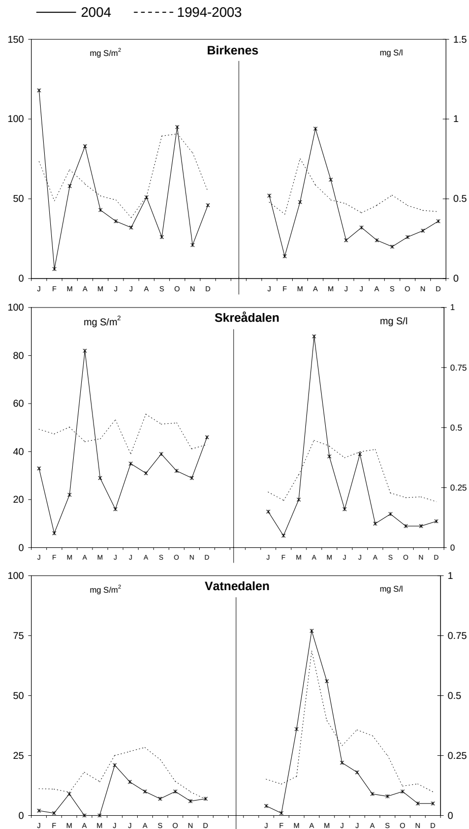
Figur 1.3: Månedlige våtavsetninger og middelkonsentrasjoner av sulfat (sjøsaltkorrigert) på norske bakgrunnsstasjoner i 2004 og de ti foregående årene (middelverdi).
