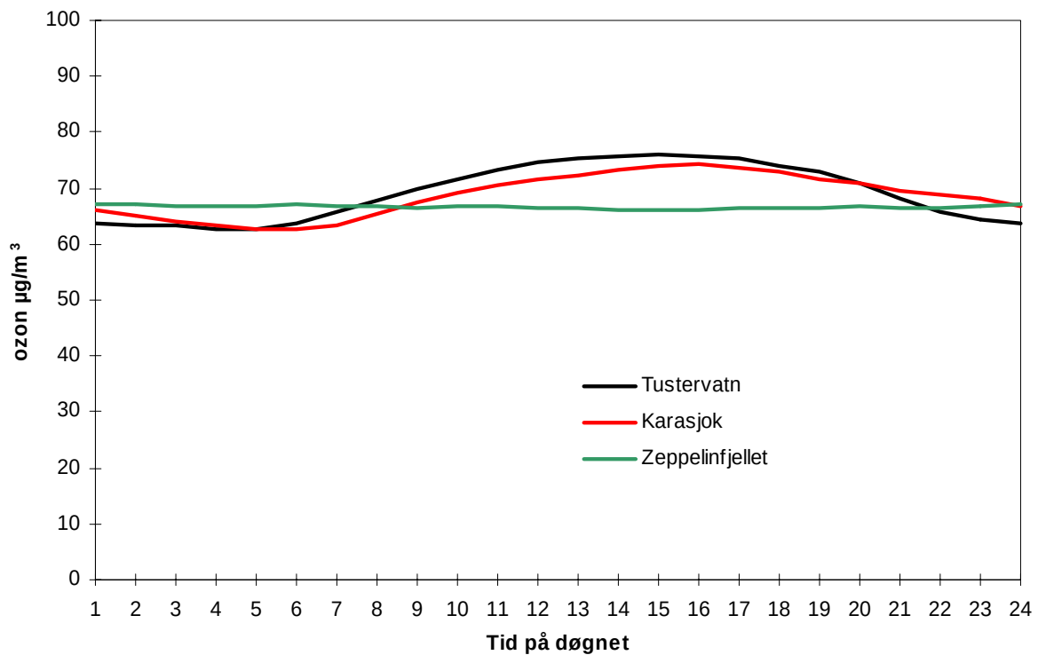
Figur 4.6: Midlere døgnvariasjon av ozon ( \mu\text{g}/\text{m}^3 ) for Tustervatn, Karasjok og Zeppelinfjellet, april-september 2004.
