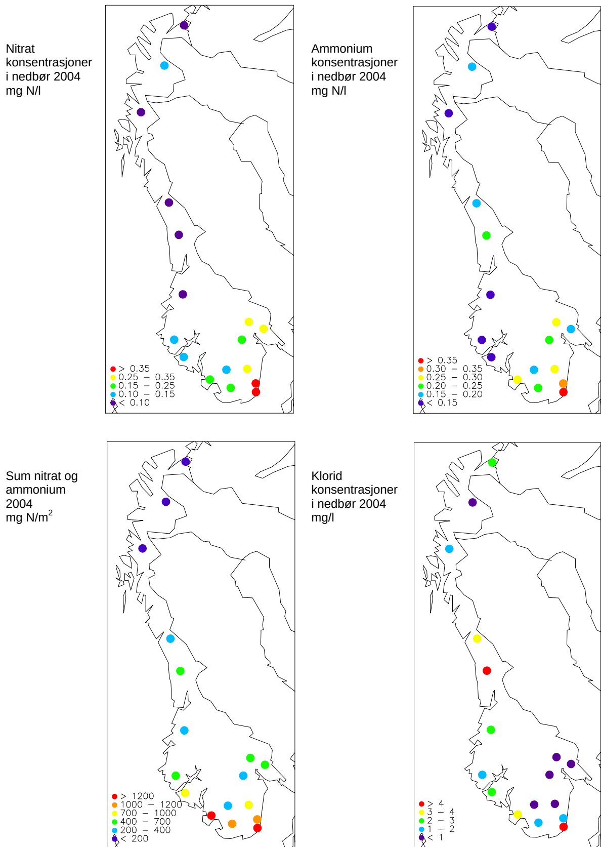
Figur 1.2: Middelkonsentrasjoner i nedbør av nitrat, ammonium og klorid, og våtavsetning av total nitrogen (nitrat + ammonium) på norske bakgrunnsstasjoner i 2004.
