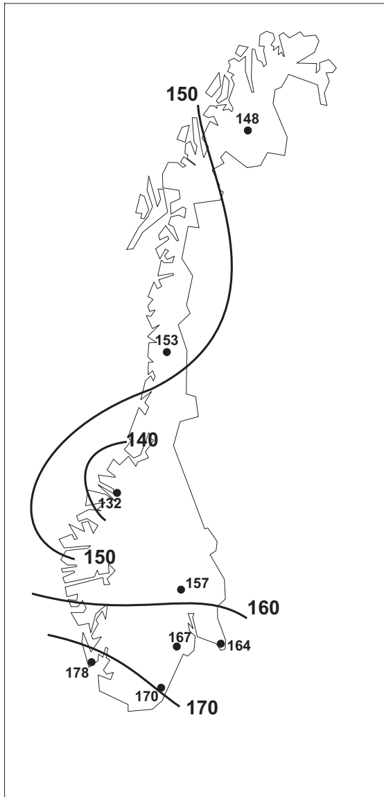
Figur 4.8: Antall døgn med 8-timers middelerdi av ozon over 60 \mu\text{g}/\text{m}^3 , april–september 2004.
