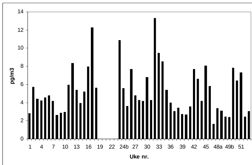
Figur 5.8: Ukentlig luftkonsentrasjon av sum PCB på Birkenes i år 2004.
