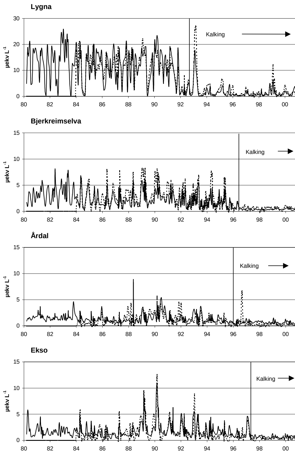
Figur 37. Enkeltobservasjoner av H + og LAl. Tidsperiode for start av kalking er indikert med strek. Stiplet linje er Al m+ , heltrukken linje er H + (NB! Forskjellig skala på figurene). Enheten er i \mu\text{ekv L}^{-1} . 20 \mu\text{ekv L}^{-1} = \text{pH } 4,5 , 10 \mu\text{ekv L}^{-1} = \text{pH } 5 , 1 \mu\text{ekv L}^{-1} = \text{pH } 6 .
