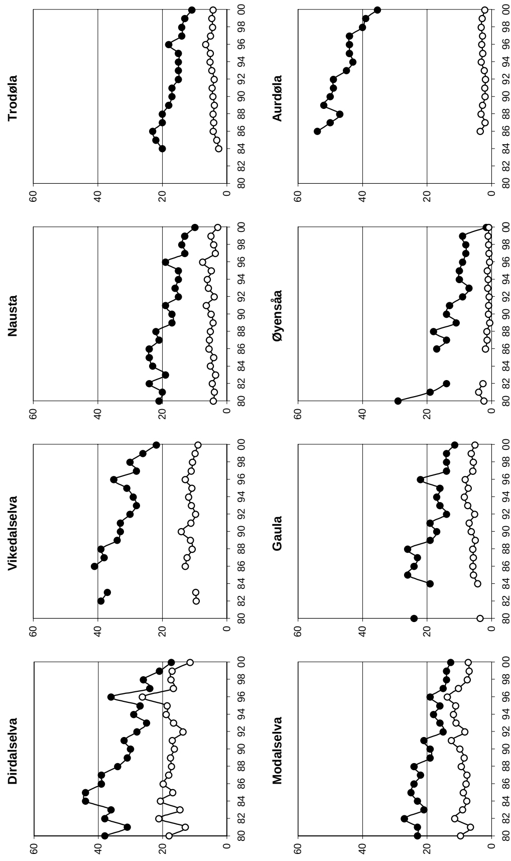
Figur 26. Ikke-marin sulfat og nitrat i ukalka elver. Ikke-marin sulfat ● og nitrat ○. Enhet \mu\text{ekv L}^{-1} .
