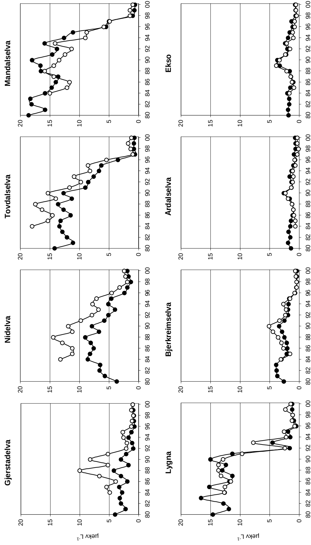
Figur 33. H^+ og labilt Al i kalka elver. H^+ ● og labilt Al ○. Enhet: \mu\text{ekv L}^{-1}
