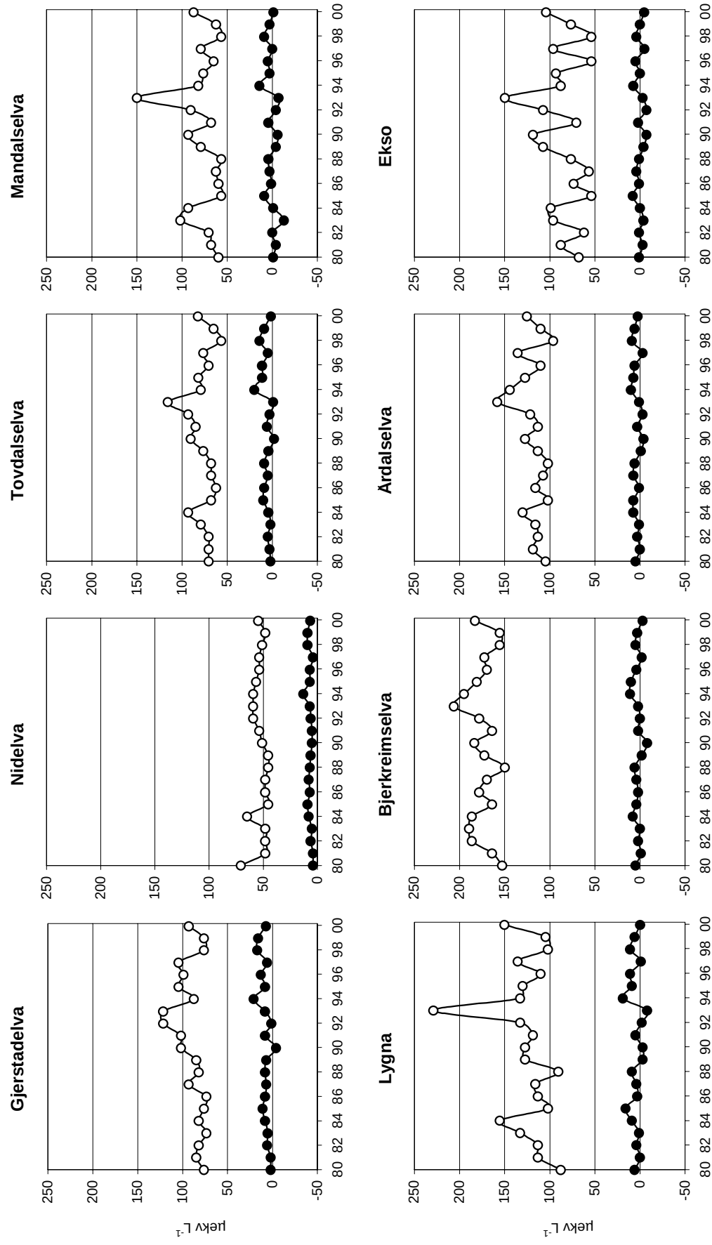
Figur 34. Klorid og ikke-marin natrium i kalka elver. Ikke-marin natrium ● og klorid ○. Enhet: \mu\text{ekv L}^{-1}
