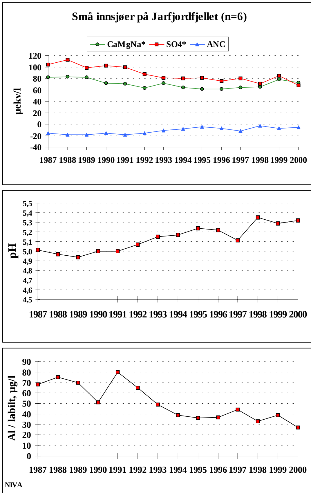
Figur 24. Forsuringsparametre for seks småvann på Jarfjordfjellet i 1987-2000. Middelverdier for basekationer, sulfat (SO4*), ANC, pH og labilt aluminium.
