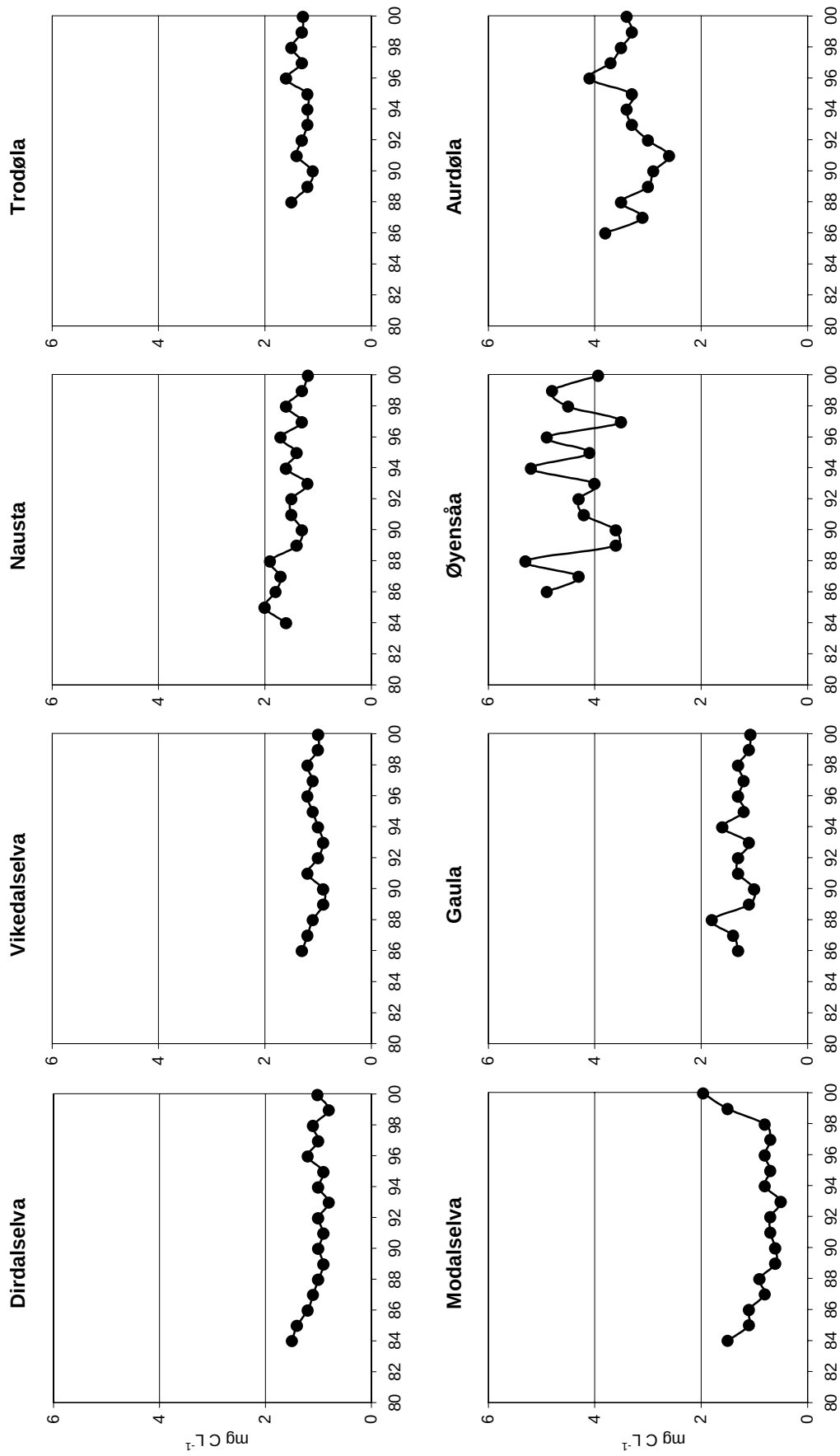
Figur 30. Total organisk karbon (TOC) i ukalka elver. Enhhet: mg CL -1
