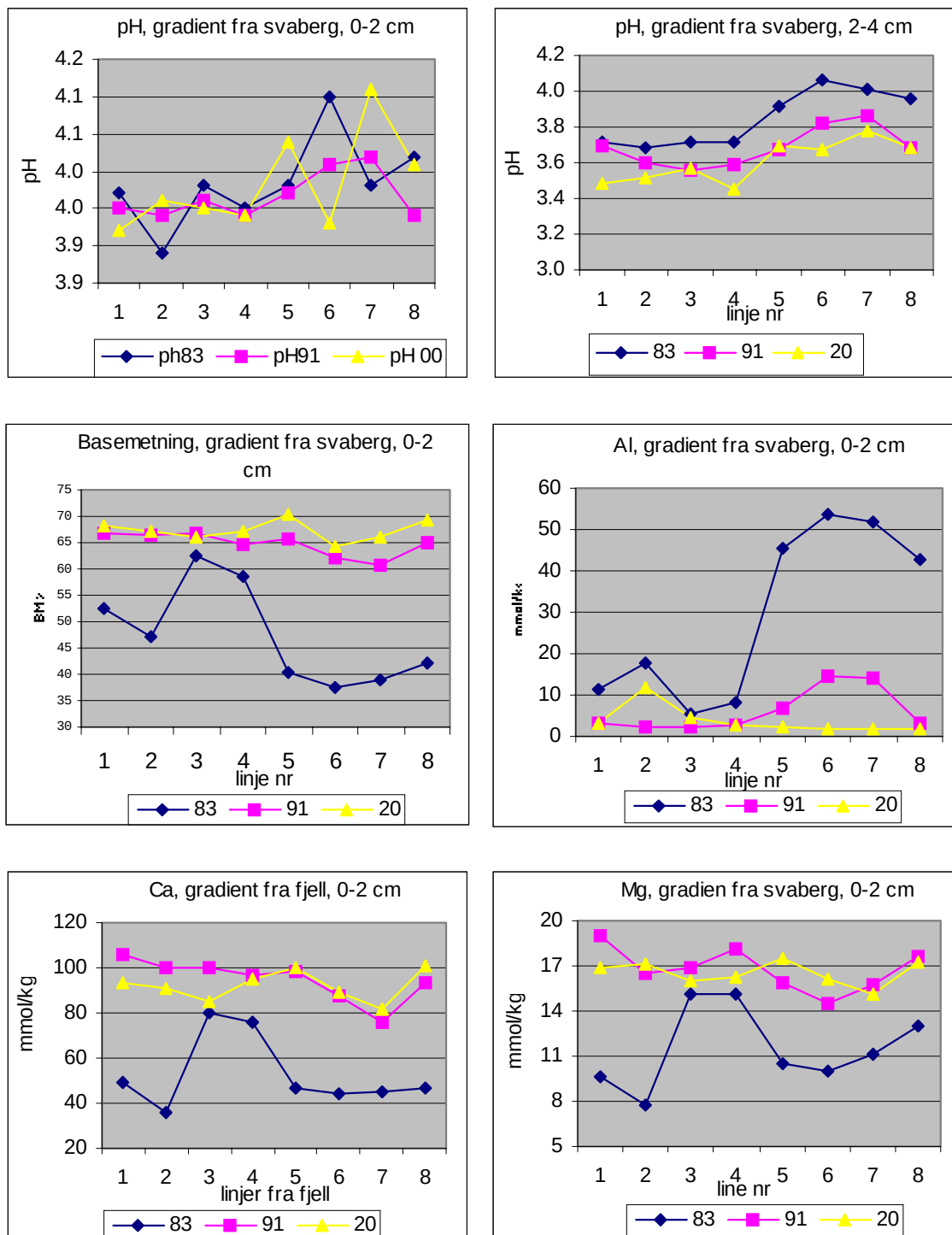
Figur 45. Utbyttbar Ca, Mg, Al, og basemetning i 0 – 2 cm dybde og pH i 0-2 og 2-4 cm i ulike avstander fra svaberg/fjell, delfelt L2 i 1983, 1991 og 2000 (83, 91 og 20). Feltets lengde er 12 – 13 m. Prøvene er tatt i åtte parallelle linjer med start ca 1 m fra svaberg/fjell og avstand på vel 1,5 m mellom linjene.
