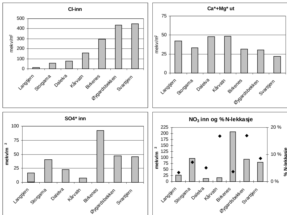
Figur 43. Beregnet total tilførsel av sjøsalter ( \text{Cl}^- ) og sur nedbør ( \text{SO}_4^* og \text{NO}_3 ) og fluks ut i avrenningen av forvittringskomponenter ( \text{Ca}^* + \text{Mg}^* ) og prosent lekkasje av nitrogen (♦) ved syv feltforskningsområder i 2000. Feltforskningsstasjonene er sortert etter økende ionetransport igjennom feltet.
