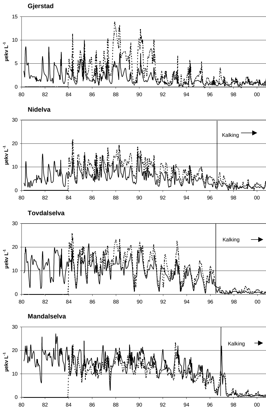
Figur 36. Enkeltobservasjoner av H^+ og LAl. Tidsperiode for start av kalking er indikert med strek. Stiplet linje er Al^{m+} , heltrukken linje er H^+ (NB! Forskjellig skala på figurene). Enheten er i \mu\text{ekv L}^{-1} . 20 \mu\text{ekv L}^{-1} = \text{pH } 4,5 , 10 \mu\text{ekv L}^{-1} = \text{pH } 5 , 1 \mu\text{ekv L}^{-1} = \text{pH } 6 .
