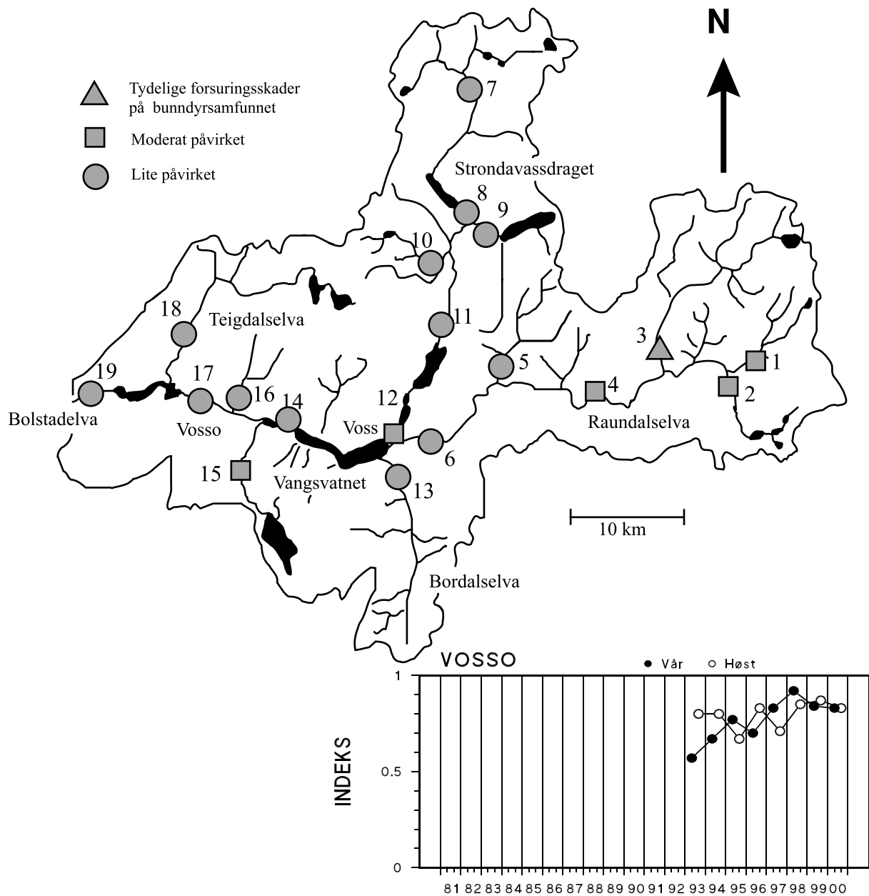
Figur 73. Oversikt over innsamlingslokaliteter og sammensetning av bunndyr i Vossovassdraget i 2000. Figuren viser også gjennomsnittlige forurensningsverdier vår (V) og høst (H) i perioden 1993-2000.
