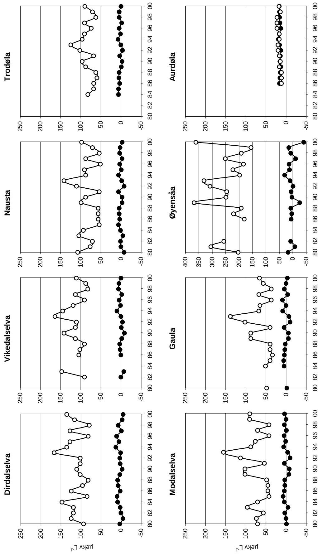
Figur 29. Klorid og ikke-marin natrium i ukalka elver. Ikke-marin natrium ● og klorid ○. Enhet: \mu\text{ekv L}^{-1}
