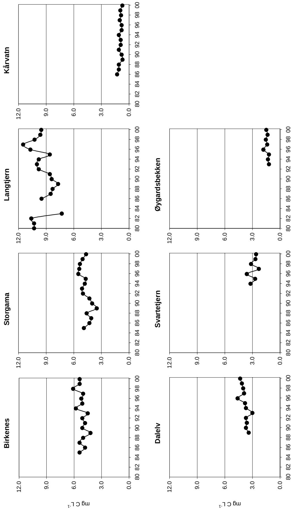
Figur 42. Total organisk karbon (TOC) i feltforskningsstasjonene. Enhet: mg C L -1
