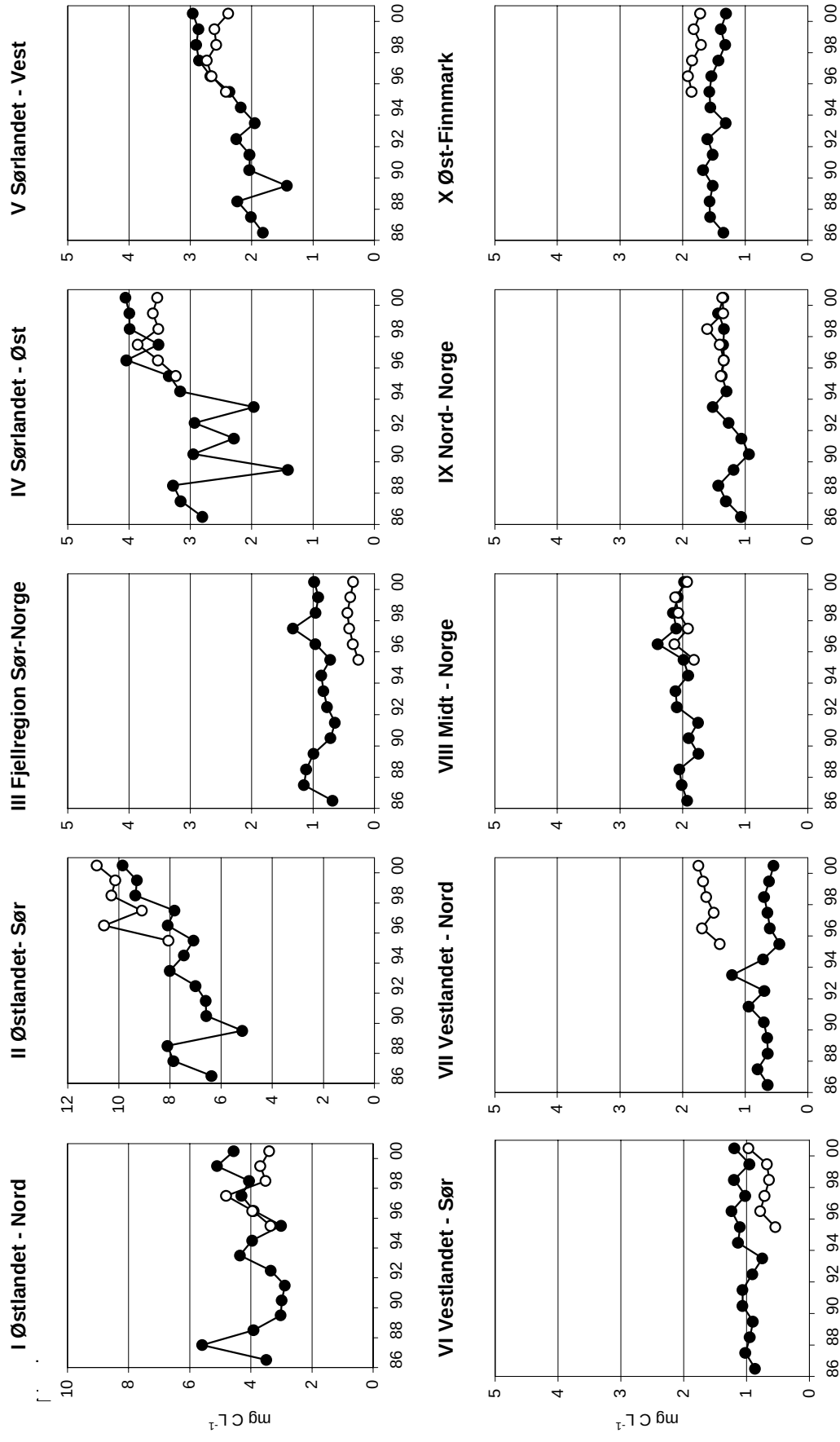
Figur 23. TOC i innsjøer – framstilt som middelvei av de undersøkte innsjøene i hver region. Lang serie (fra 1986) er ”100-sjøer” mens kort serie (fra 1995) er ”200-sjøer”. Enhet mg C L -1 .
