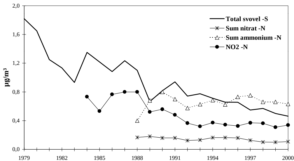
Figur 5. Midlere årlige konsentrasjoner i luft av total svovel ( \text{SO}_2 + \text{SO}_4 ), oksidert nitrogen ( \text{HNO}_3 + \text{NO}_3 ), redusert nitrogen ( \text{NH}_3 + \text{NH}_4 ) og \text{NO}_2 på norske EMEP-stasjoner ( Figur 1 ).
