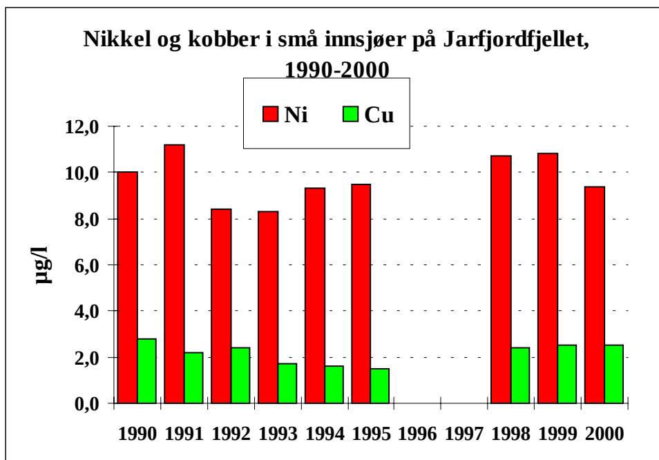
Figur 25. Nikkel og kobber i små innsjøer på Jarfjordfjellet. Årlige middelveier for seks innsjøer fra 1990 til 2000.
