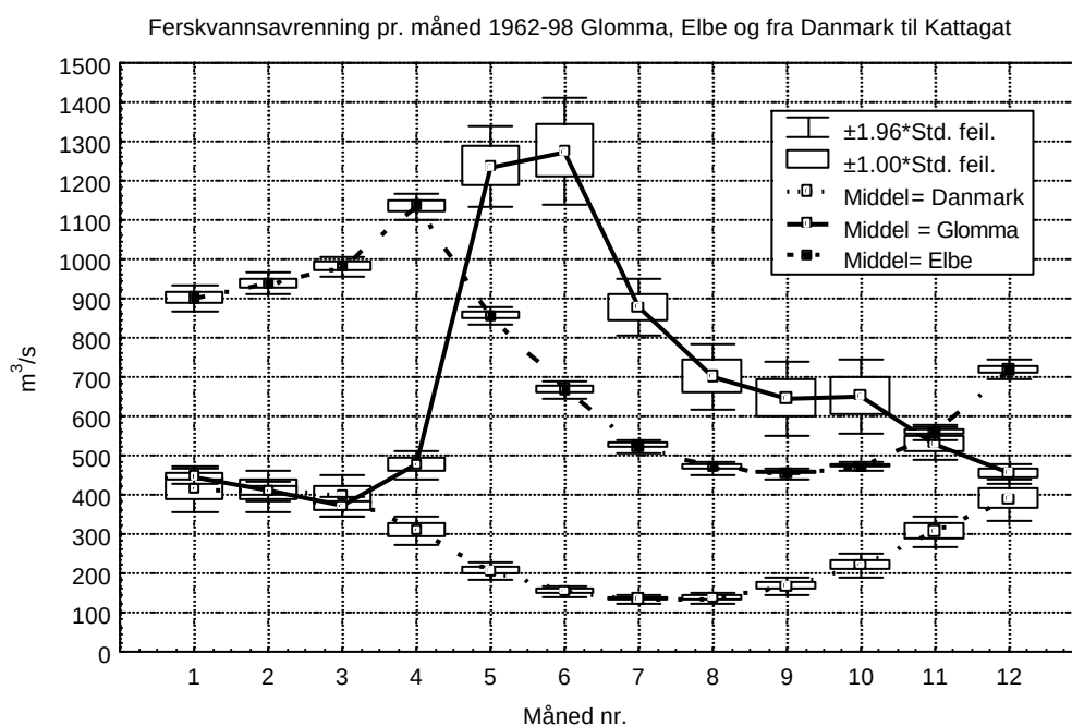
Figur 24. Vannføring (pr. måned) i Elbe, Glomma og avrenning fra Danmark til Kattegat 1962-98. Data fra Danmarks miljøundersøkelser, og Helgoland Biologiske stasjon.
