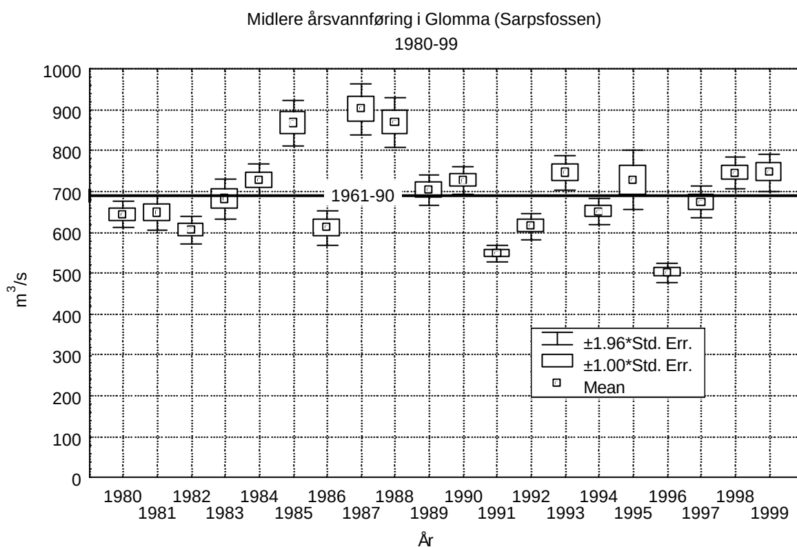
Figur 18. Årlig middelvannføring i Glomma (Sarpsfossen) 1980-99 sammenlignet med gjennomsnittet for 30-års middelverdien (1961-1990). Data fra NVE.
