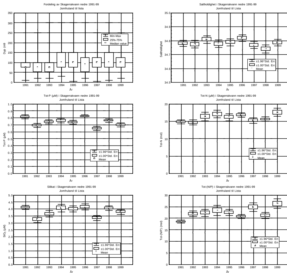
Figur 50. Skagerrakvann nedre - fordeling og årsmiddel av samtlige observasjoner av saltholdighet, tot-P, tot-N, \text{SiO}_3 og Tot- (N/P) på Jomfruland, Arendal St. 2 og 3 samt Lista i 1991-99.
