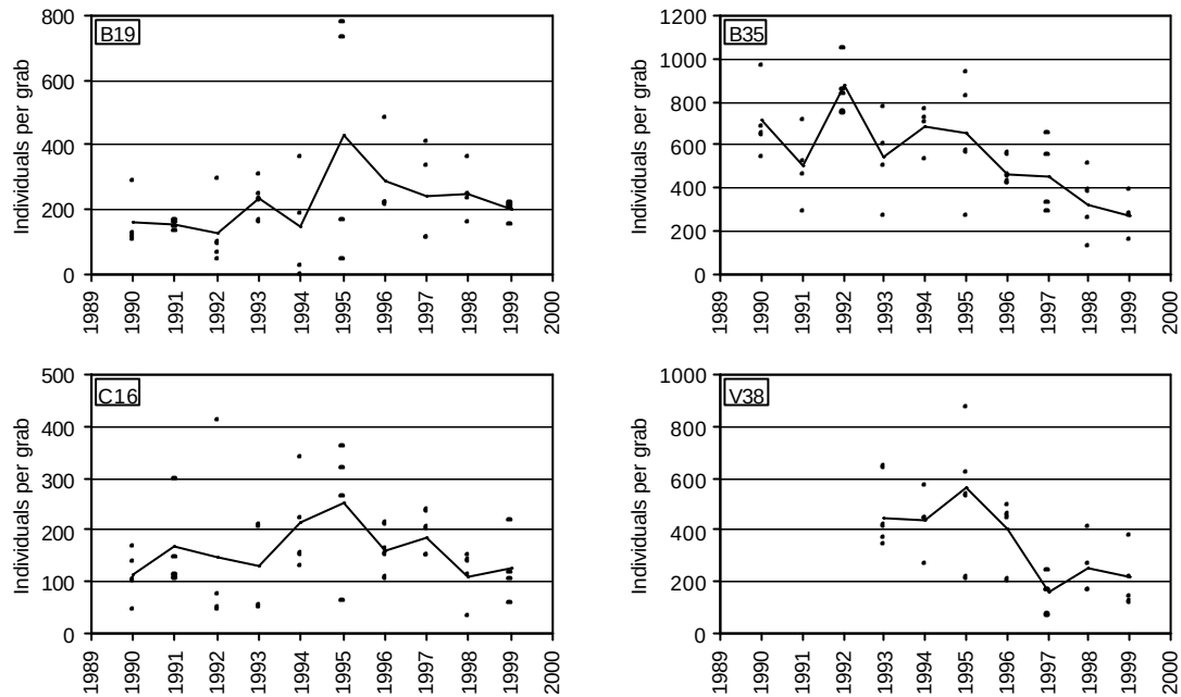
Figur 60. Individantall pr. grabb (0.1 m 2 ) (punkter) og gjennomsnitt pr. år (linjer) på utvalgte stasjoner i 1990-1999.
