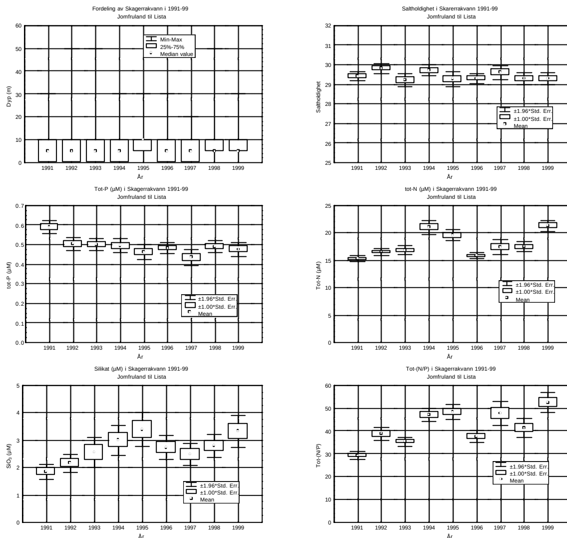
Figur 46. Skagerrak kystvann - fordeling og årsmiddel av samtlige observasjoner av saltholdighet, tot-P, tot-N, SiO 3 og Tot- (N/P) på Jomfruland, Arendal St. 2 og 3 samt Lista i 1991-99.
