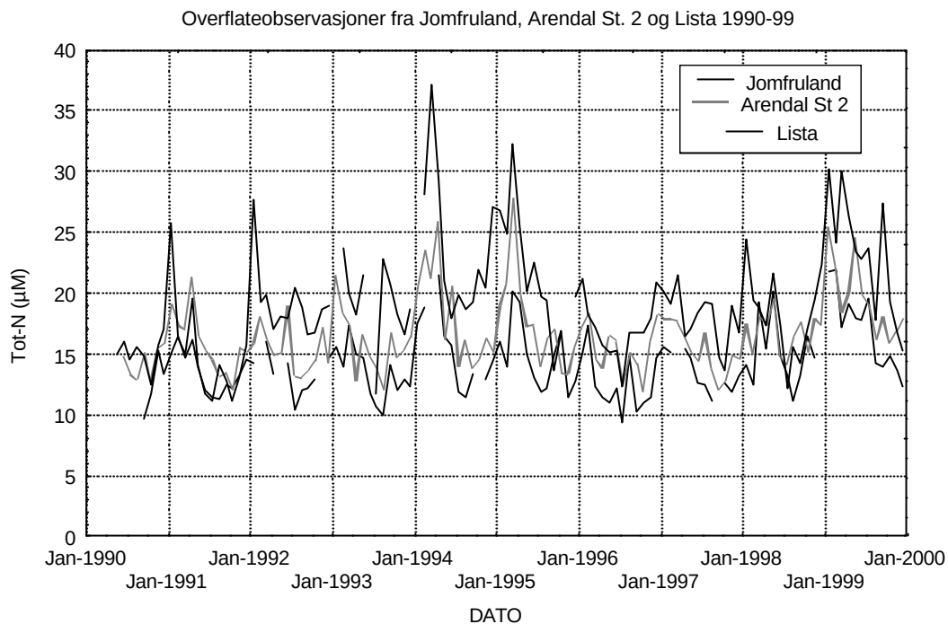
Figur 30. Tot-N, 0-10 meters dyp, 1990-99, månedsmiddel.
