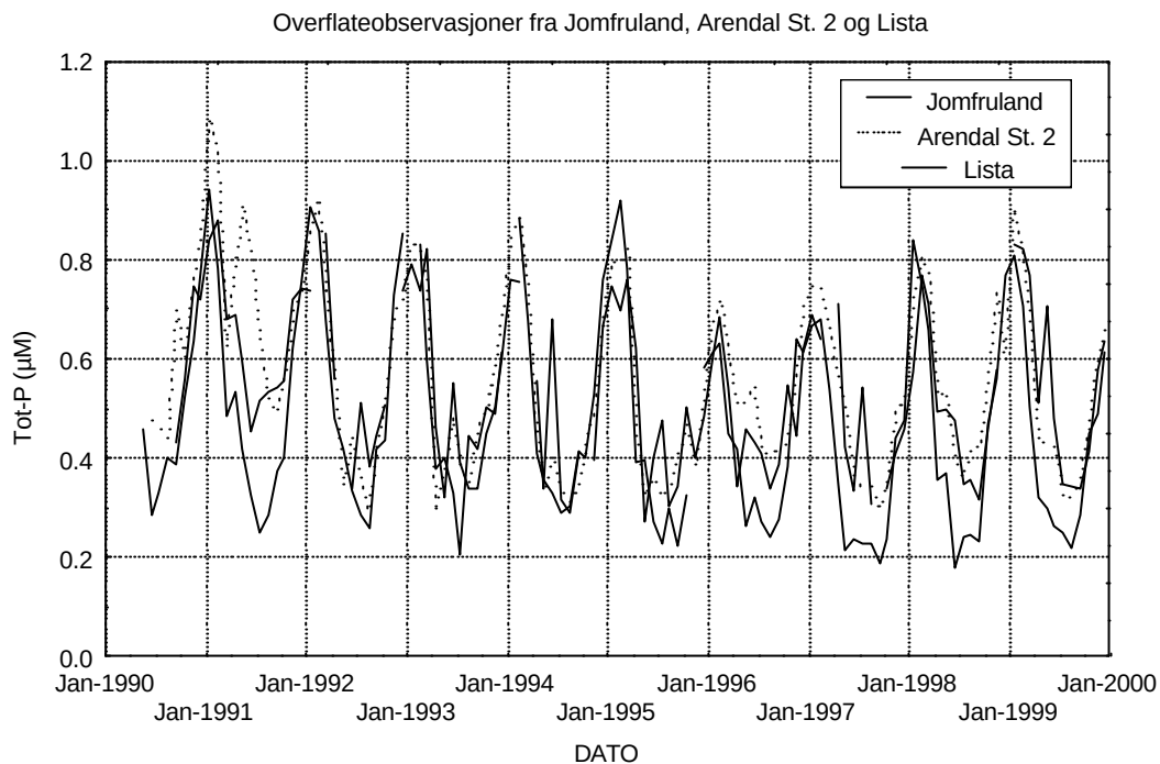
Figur 32. Tot-P, 0-10 meters dyp, 1990-99, månedsmiddel.
