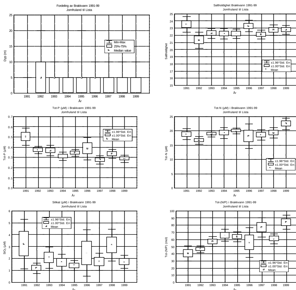
Figur 44. Fordeling og årsmiddel av samtlige observasjoner i brakkvann av saltholdighet, tot-P, tot-N, \text{SiO}_3 og Tot-(N/P) på Jomfruland, Arendal St. 2 og 3 samt Lista i 1991-99.
