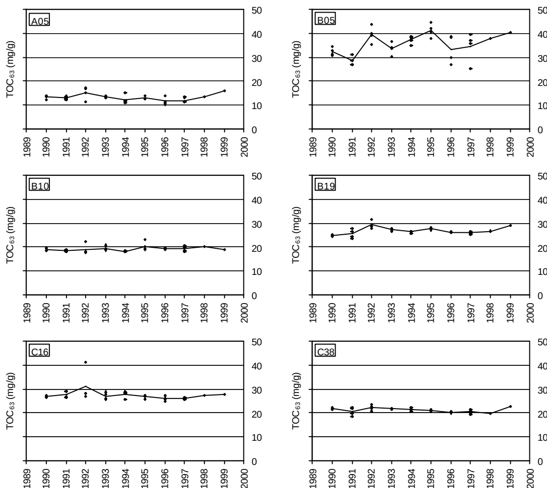
Figur 57. Innhold av totalt organisk karbon (TOC 63 , mg/g), korrigert for sedimentets innhold av silt og leire i enkeltprøver og som gjennomsnitt pr. år på utvalgte stasjoner 1990-1999
