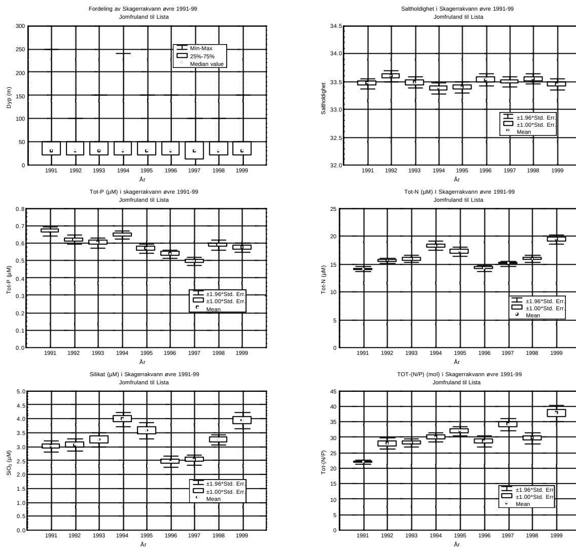
Figur 48. Skagerrakvann øvre - fordeling og årsmiddel av samtlige observasjoner av saltholdighet, tot-P, tot-N, \text{SiO}_3 og Tot- (N/P) på Jomfruland, Arendal St. 2 og 3 samt Lista i 1991-99.
