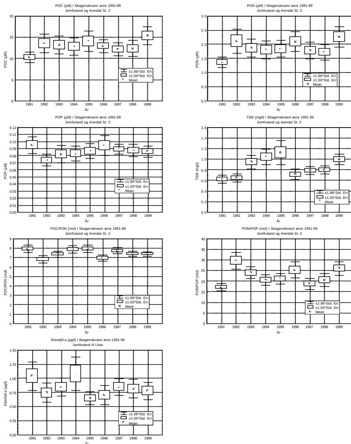
Figur 49. Årsmiddel i Skagerrakvann øvre av partikulært organisk bundet karbon (POC), nitrogen (PON) og fosfor (POP), C/N- og N/P-forhold samt totalt suspendert materiale (TSM) ved Jomfruland og Arendal St. 2, samt klorofyll- a ved Jomfruland til Lista 1991-99.
