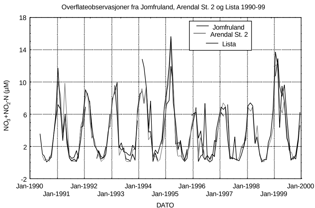
Figur 31. Nitrat+nitritt, 0-10 meters dyp 1990-99, månedsmiddel.
