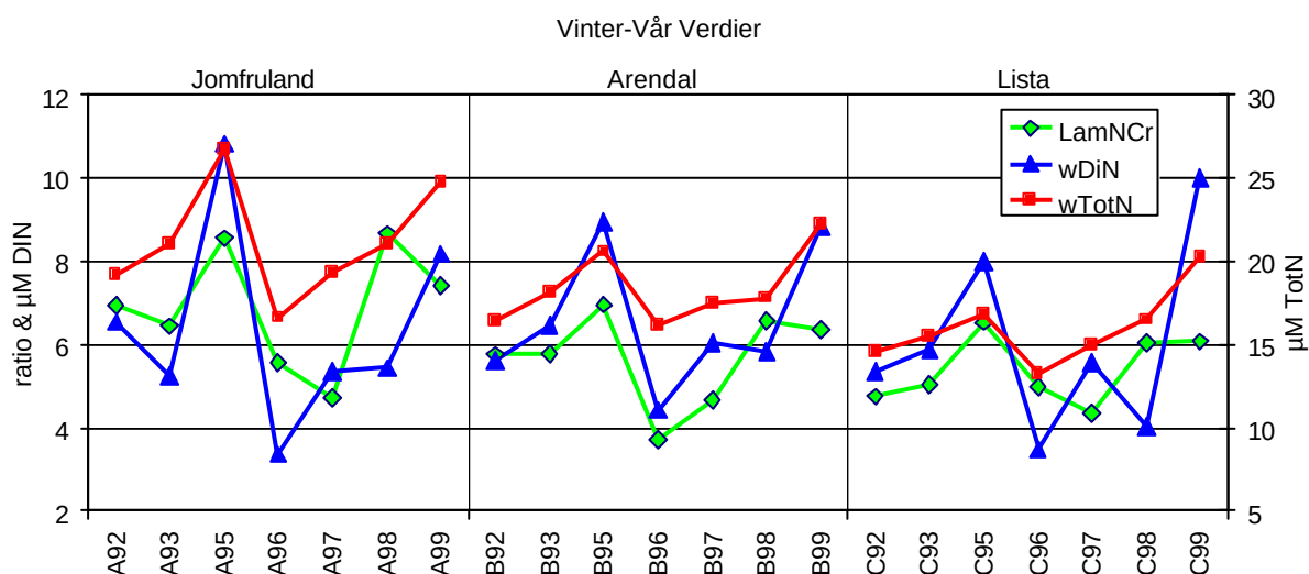
Figur 70. Nitrogen/karbon-ratio (gjennomsnitt av 4 stasjoner i hver region: A, B og C) i lamina av stortare (LamNCr, ruter) plottet sammen med vinterkonsentrasjoner av DIN ( \text{wDiN} = \text{NO}_3 + \text{NO}_2 + \text{NH}_4 ) og tot-N ( \text{wTotN} ) i sjøvannet (gjennomsnitt desember-mai, 0-10m dyp) i tidsperioden 1992-1999.
