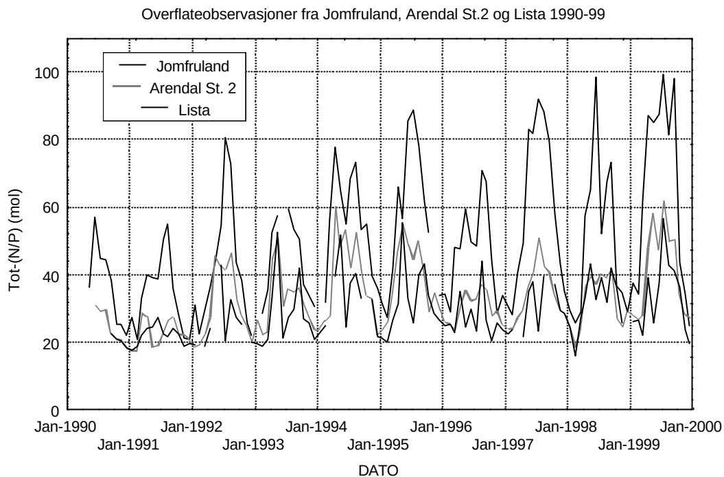
Figur 34. Tot-(N/P), 0-10 meters dyp, 1990-99, månedsmiddel.
