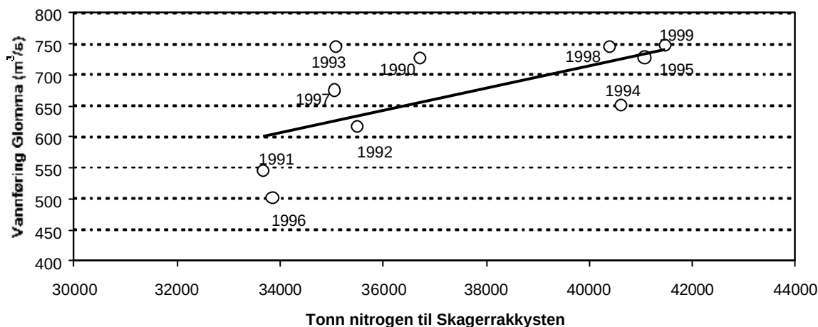
Figur 19. Årlig middelvannføring i Glomma og totaltilførsler av nitrogen fra Norge til Skagerrakkysten.
