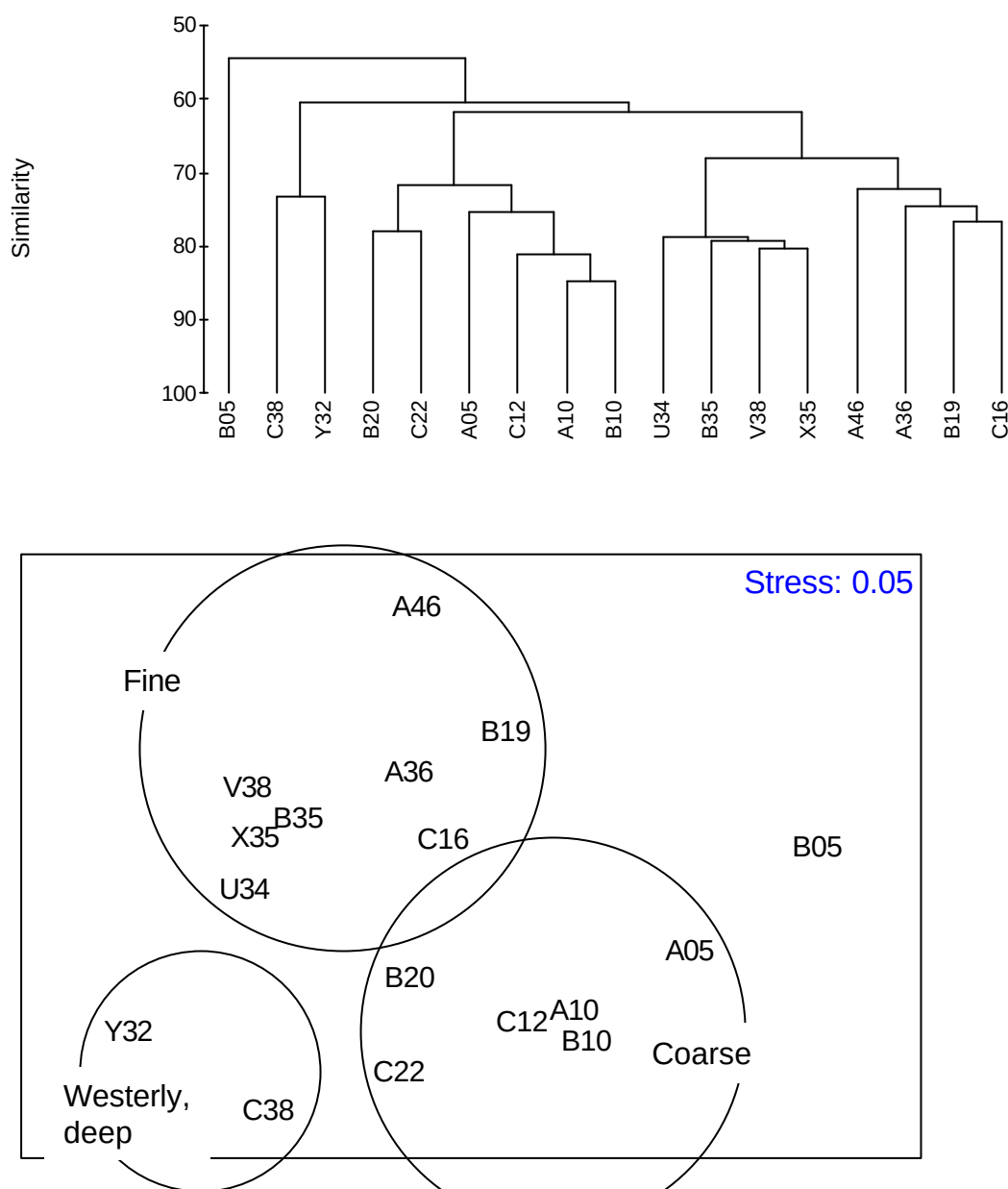
Figur 77. Cluster-dendrogram og MDS-plott av likheter blant 17 stasjoner, aggregert 1990-1999. Innsirklede stasjoner illustrerer stasjonsgrupper fremkommet ved 65% likhetsnivå i cluster-analysen. Gruppene korresponderer stort sett med sedimentkarakteristika og geografisk beliggenhet av stasjonene.
