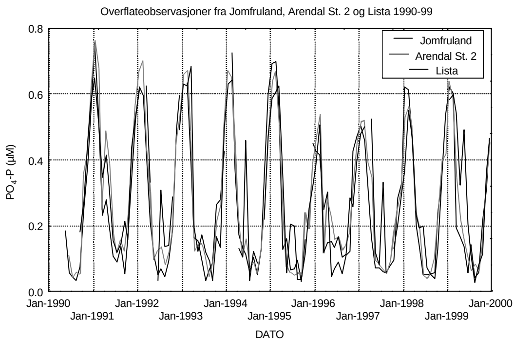
Figur 33. Fosfat, 0-10 meters dyp, 1990-99, månedsmiddel.
