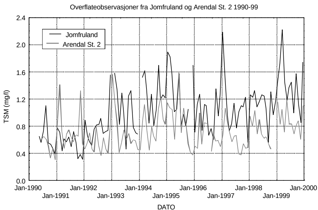
Figur 35. TSM, 0-10 meters dyp, 1990-99, månedsmiddel.
