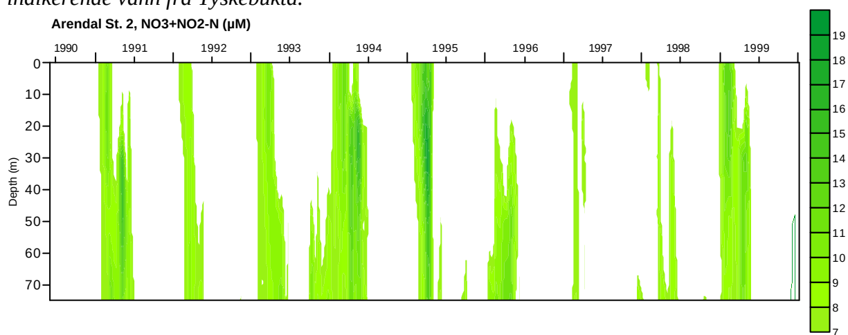
Figur 23. Nitrat+nitrit (µM) ved st. Arendal 2 1990-99, bare konsentrasjoner over 7 (µM) er markert.
